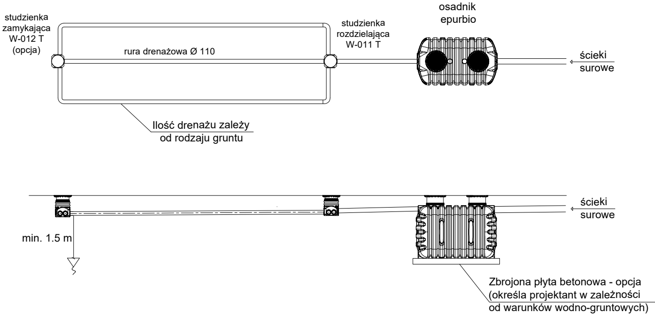
Przykładowy rzut i przekrój osadnika epurbio z drenażem rozsączającym
