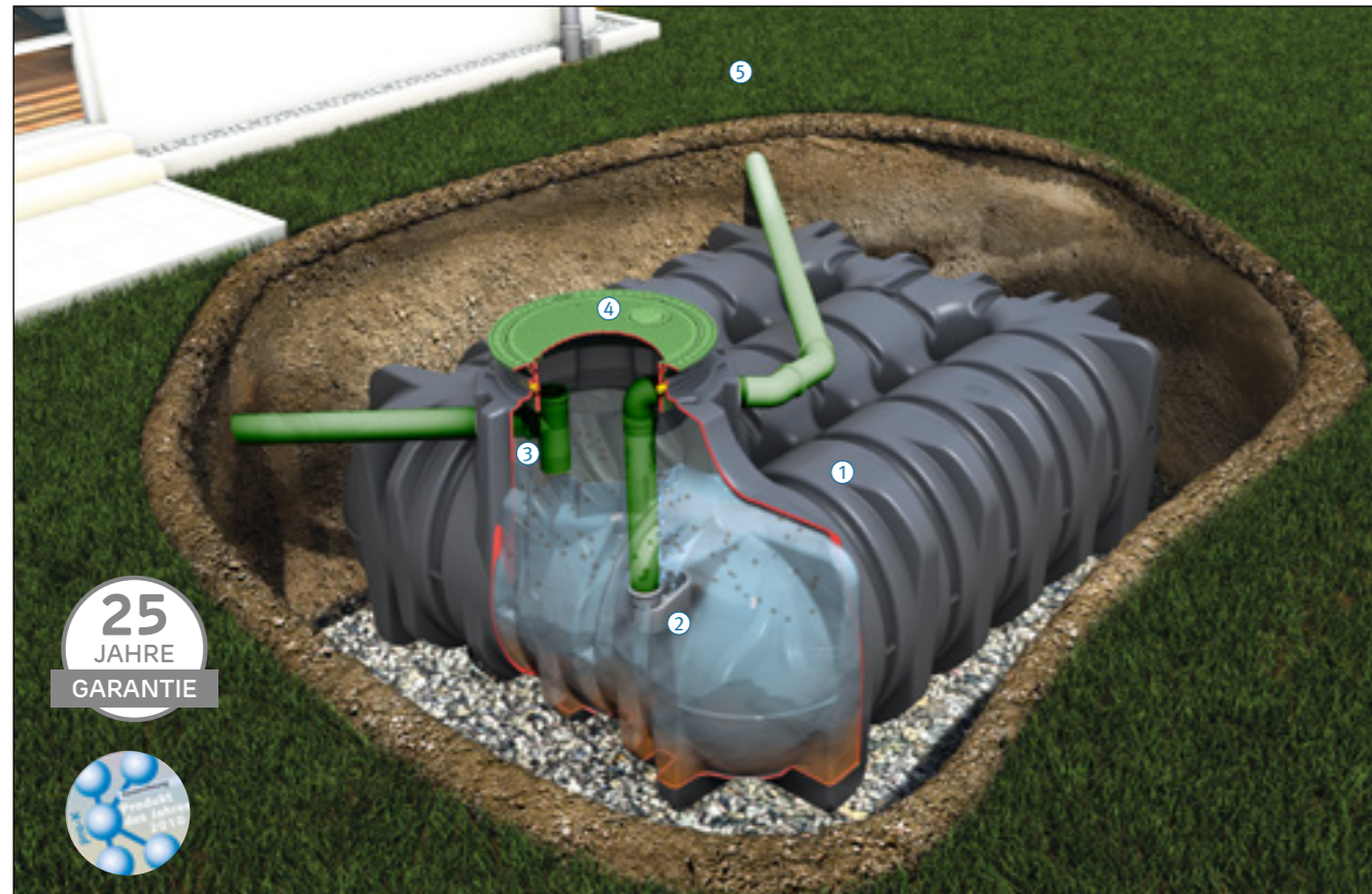
Abbildung zeigt Flachtank Platin M 153 Sedimentationstank mit Lieferumfang und Teleskop-Domschacht Mini (Zubehör)
