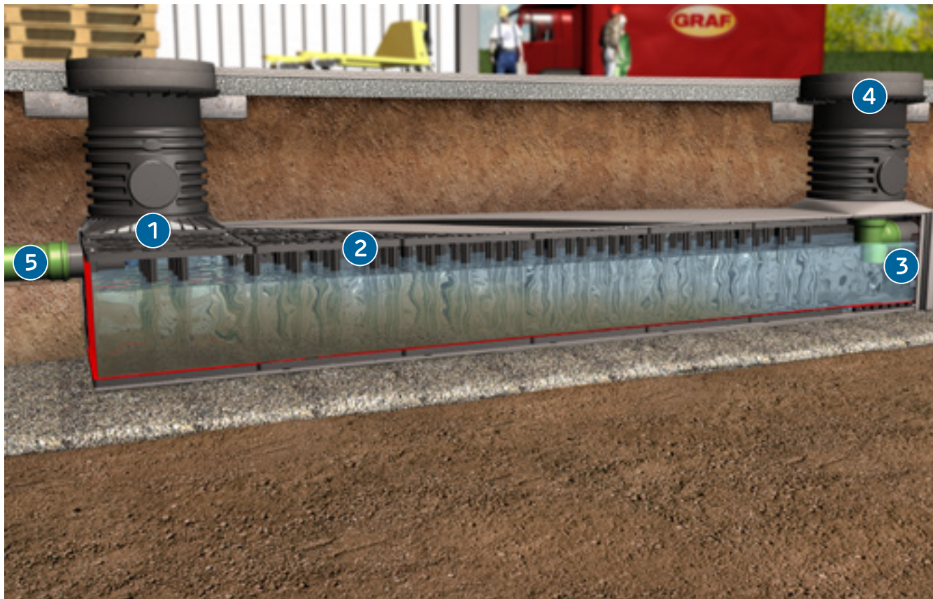
Abbildung zeigt Vario 800 – EcoBloc Sedimentationstank (Zubehör ab Seite 76)
