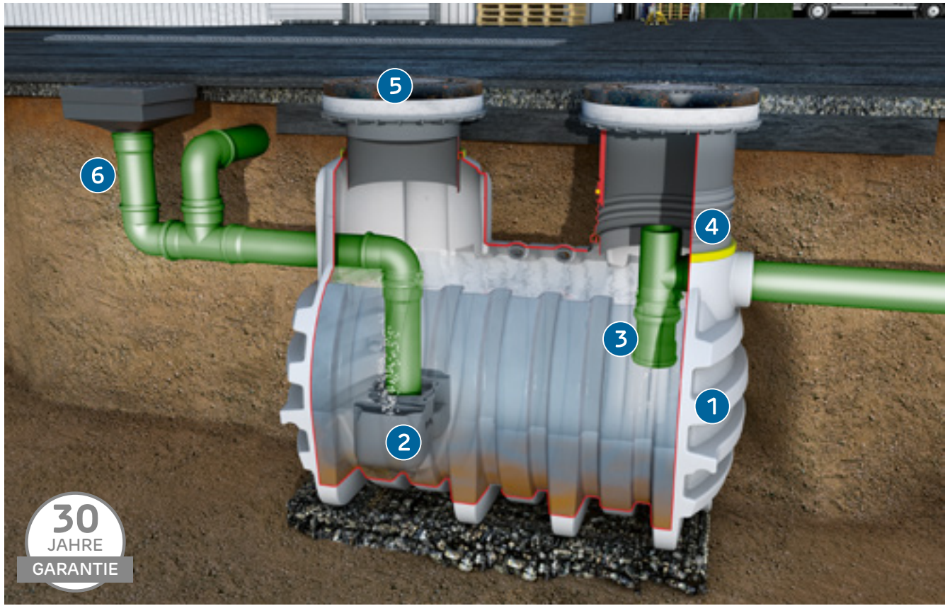
Abb. zeigt Erdtank Diamant Sedimentationstank mit Lieferumfang und 2 x Teleskop-Domschacht 600 (Zubehör ab Seite 76), 2 x Betonabdeckung und Lastverteilerplatte (bauseits)
