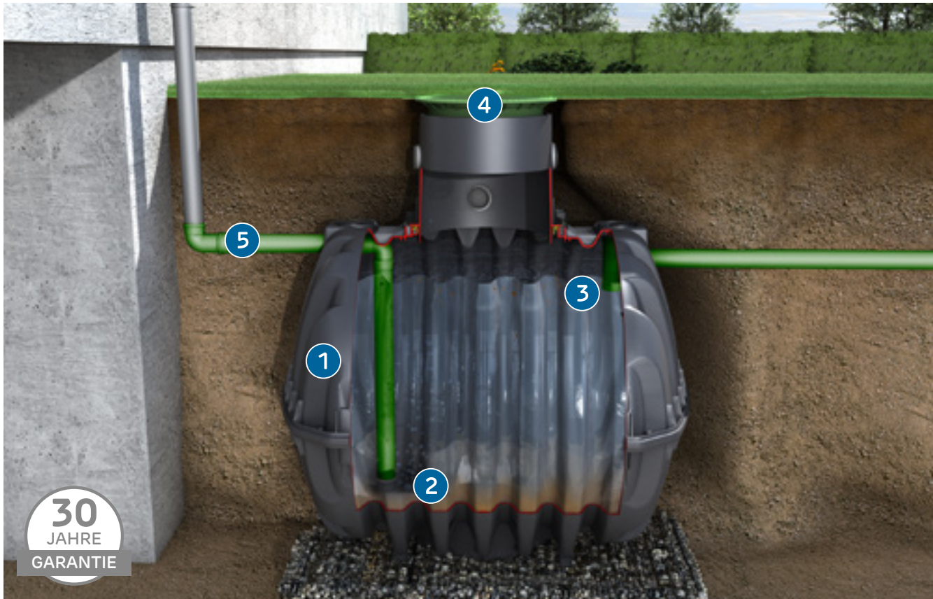
Abb. zeigt Erdtank Carat Sedimentationstank mit Lieferumfang und Teleskop-Domschacht 600 Mini (Zubehör ab Seite 76)
