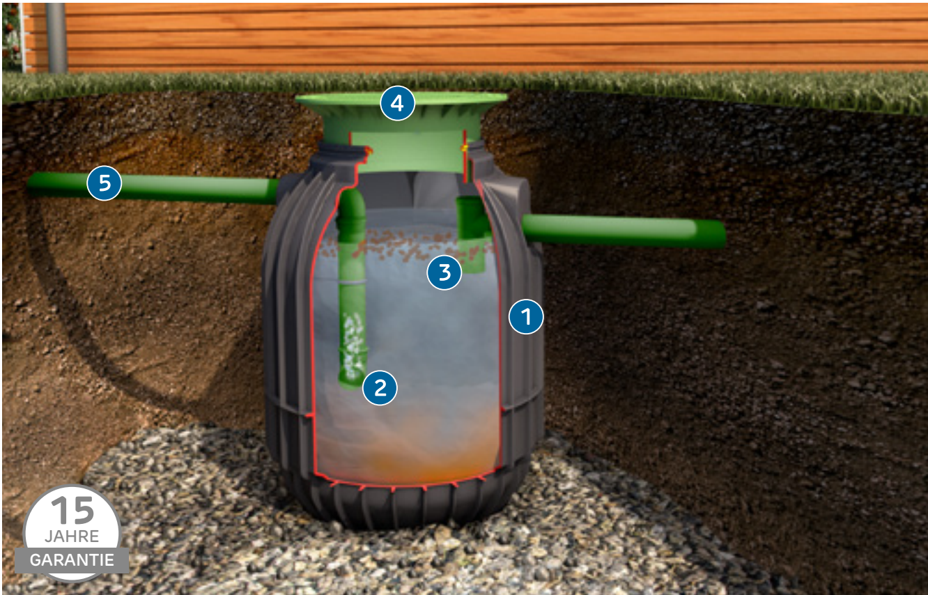
Abbildung zeigt Saphir Sedimentationstank mit Lieferumfang und Teleskop-Domschacht 600 Mini (Zubehör Seite 76)
