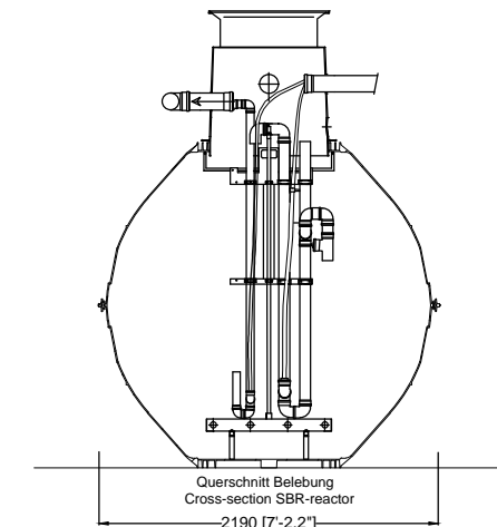
C - C
