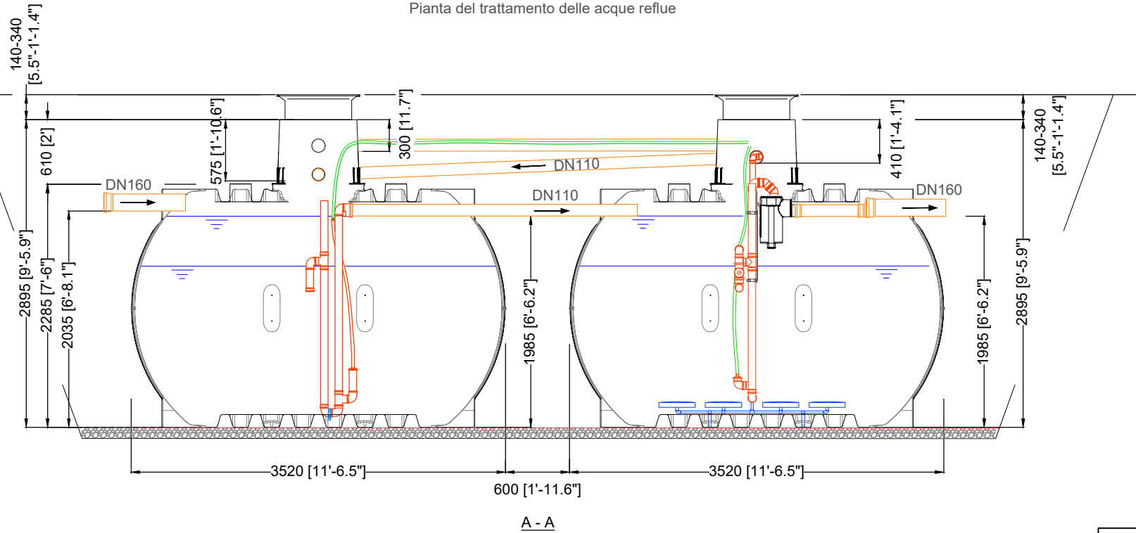
Grundriss Abwasserbehandlung Top view wastewater treatment Plan de mise en oeuvre Planta tratamiento de aguas residuales Pianta del trattamento delle acque reflue
