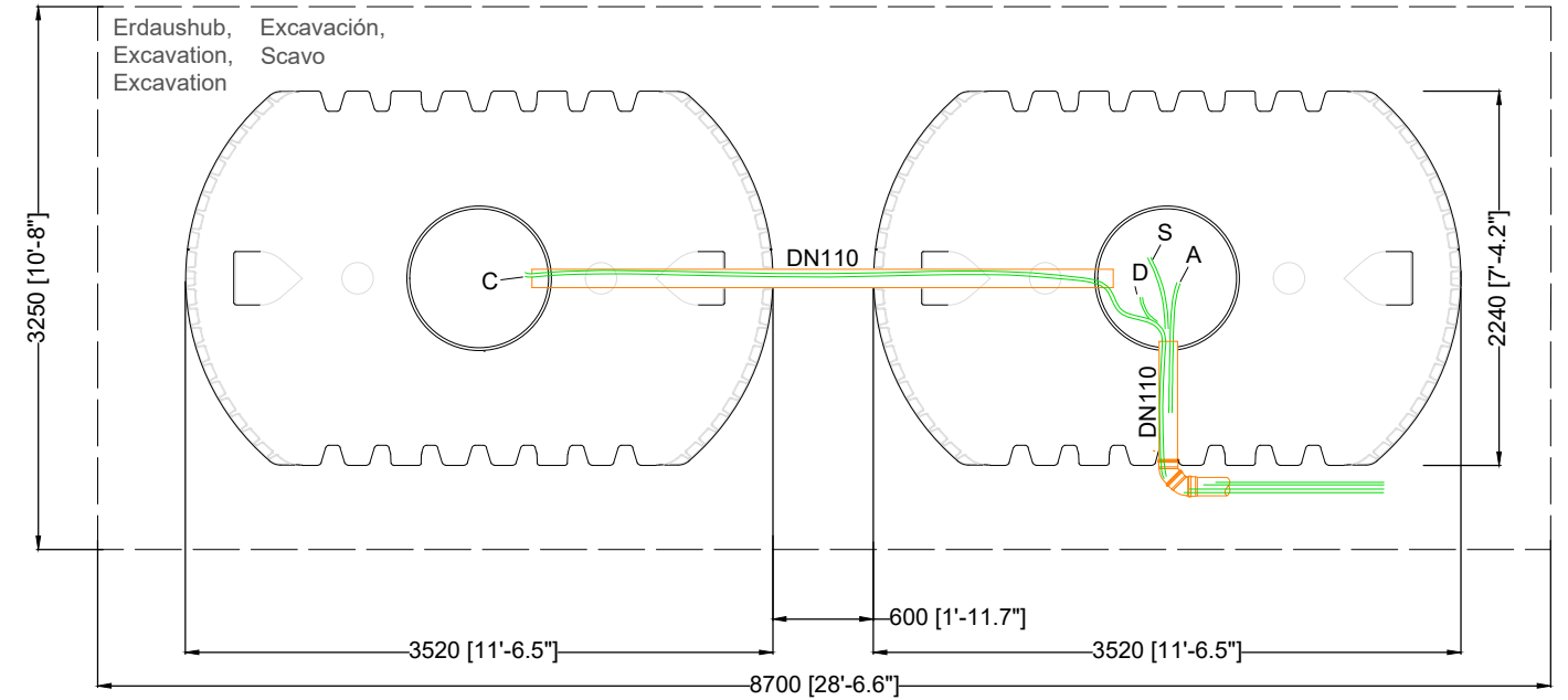
Grundriss Luftschläuche Top view compressed air Plan de raccordement des tuyaux d'air Vista superior tubería aire comprimido Pianta dei tubi di aria compressa
