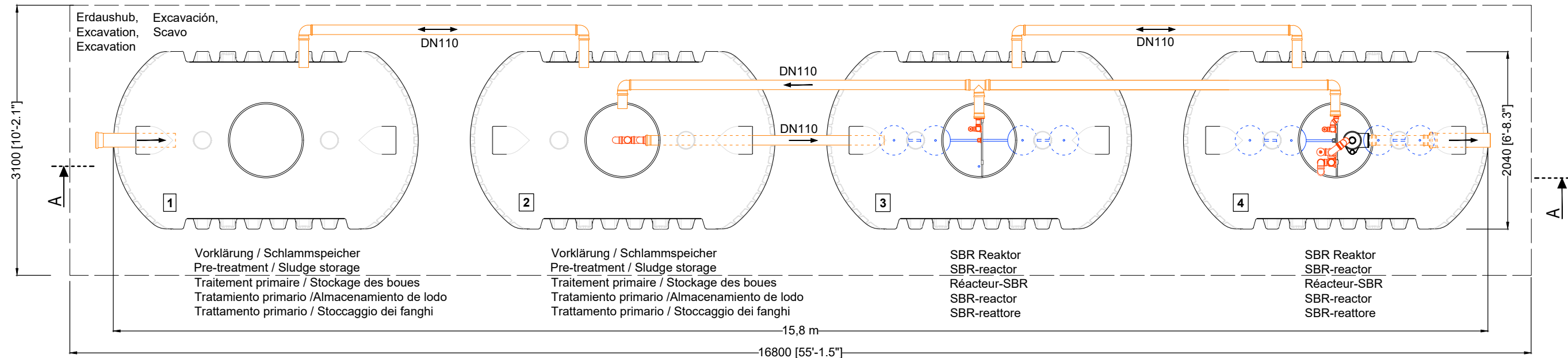
Grundriss Abwasserbehandlung Top view wastewater treatment Plan de mise en oeuvre Planta tratamiento de aguas residuales Pianta del trattamento delle acque reflue
