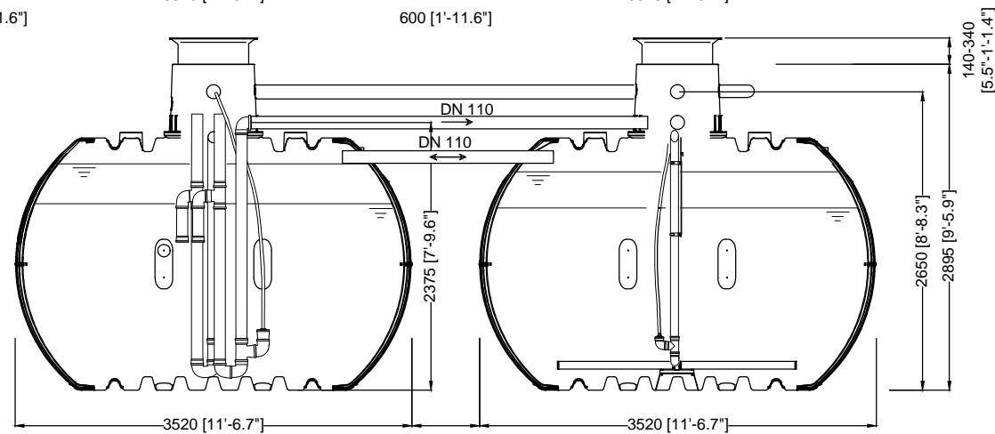
Schnitt B-B
