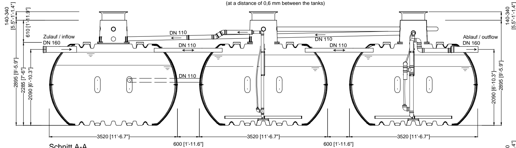
Schnitt A-A
