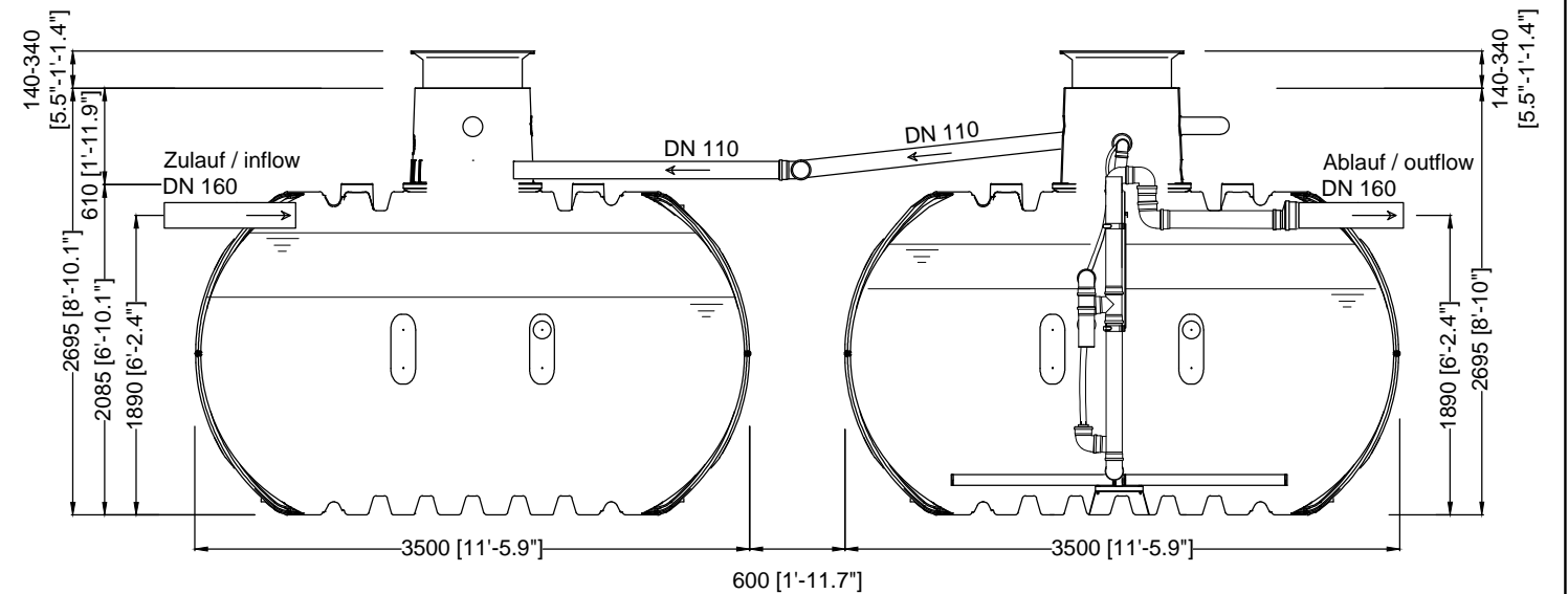
Schnitt B-B
