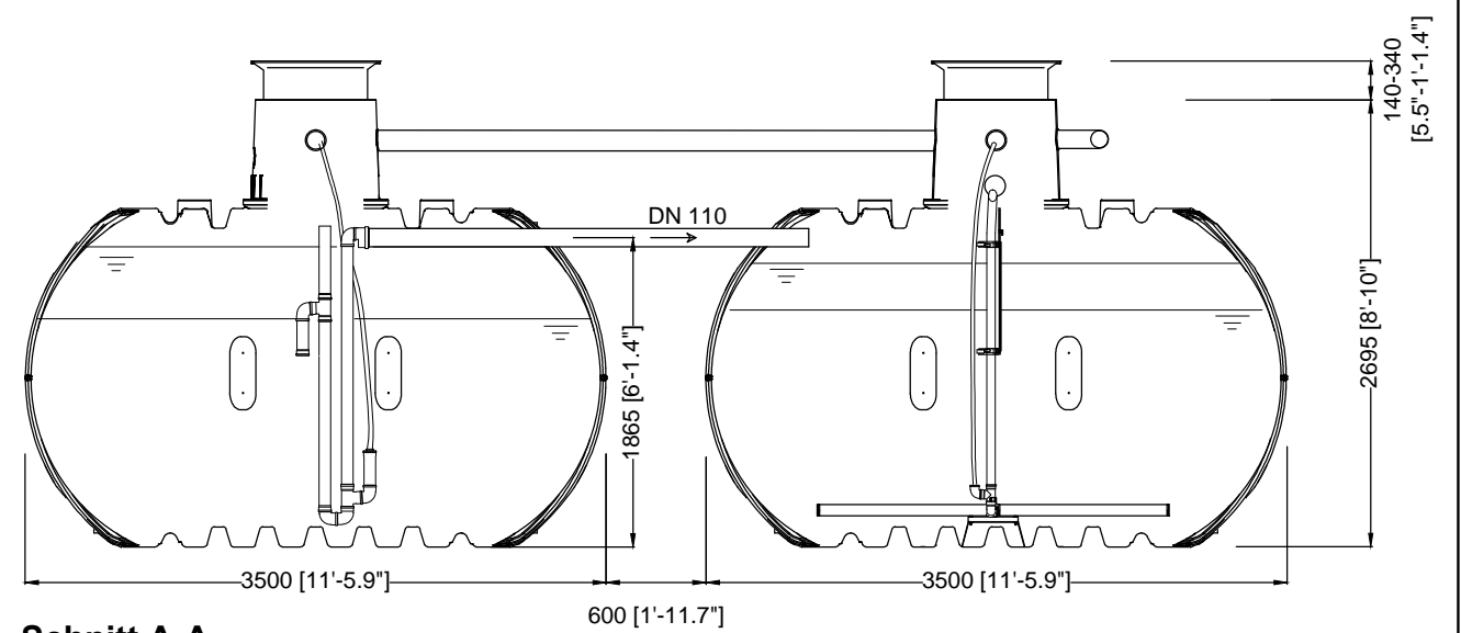
Schnitt A-A
