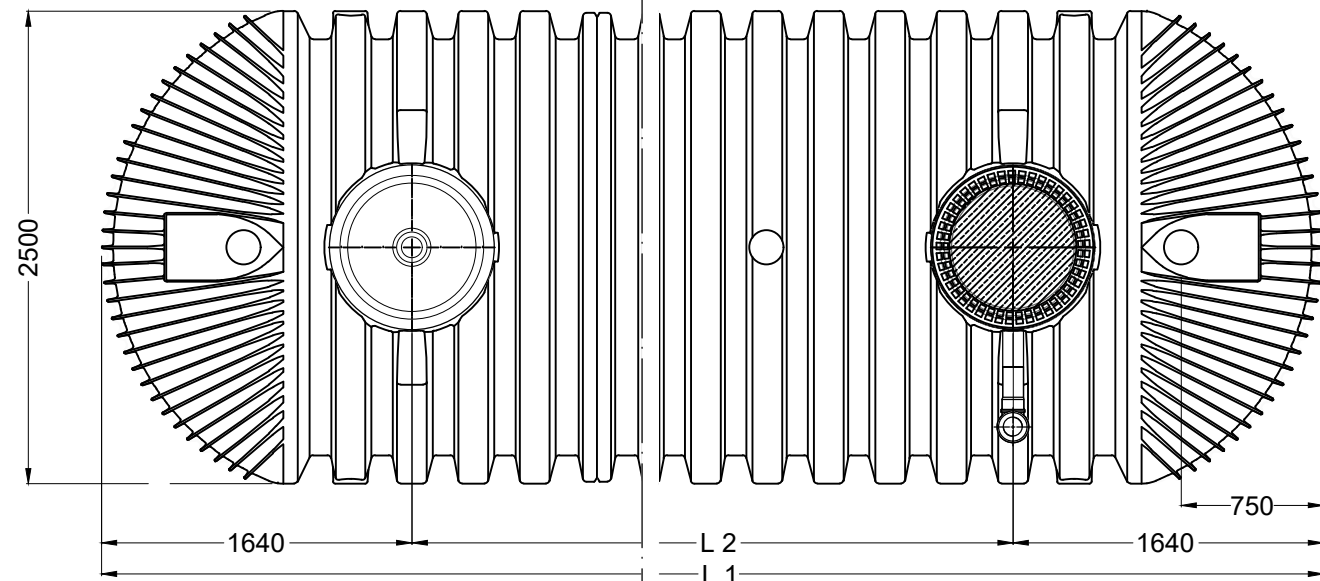
Tankanlage LKW befahrbar SLW 40 bei Erdüberdeckung 1000 -1500 mm
