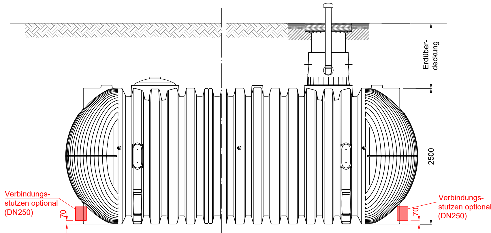
Tankanlage LKW befahrbar SLW 40 bei Erdüberdeckung 1000 -1500 mm
