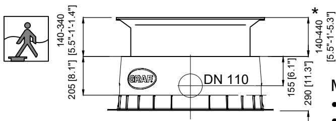
A-A
