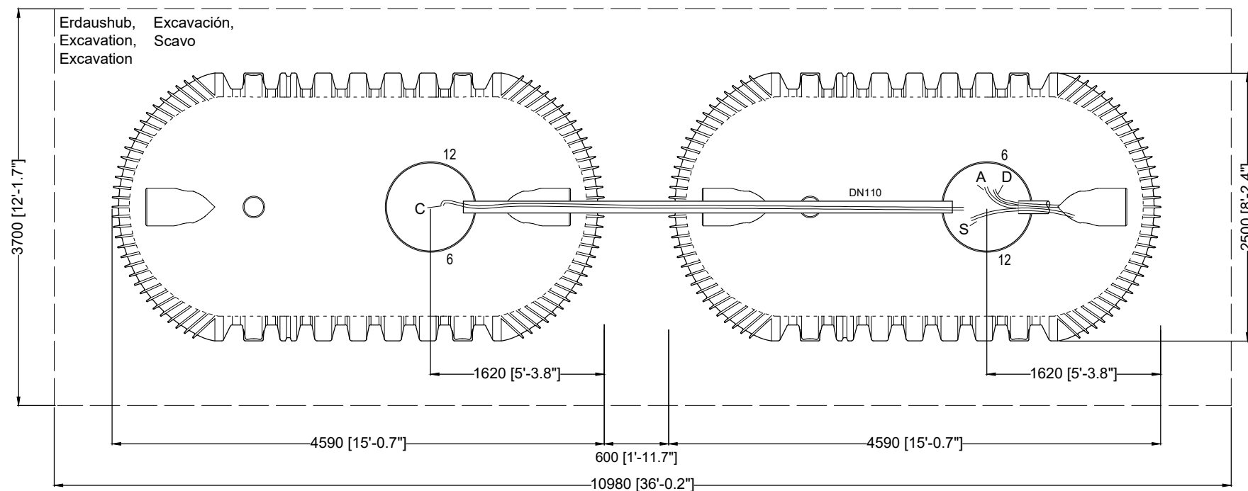
Grundriss Luftschläuche Top view compressed air Plan de raccordement des tuyaux d'air Vista superior tubería aire comprimido Pianta dei tubi di aria compressa
