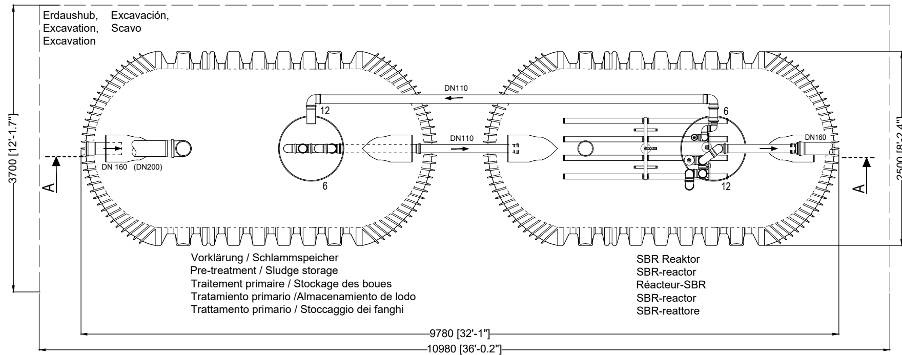
Grundriss Abwasserbehandlung Top view wastewater treatment Plan de mise en oeuvre Planta tratamiento de aguas residuales Pianta del trattamento delle acque reflue
