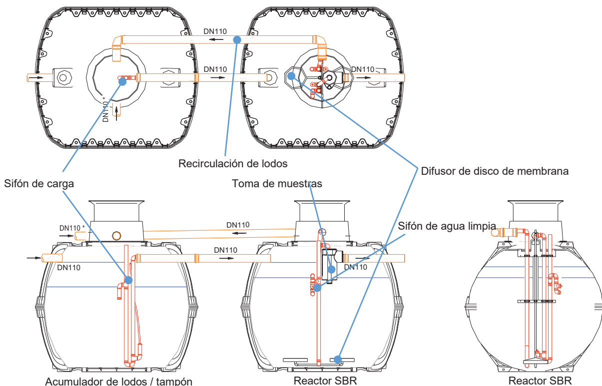
Imagen 4: Ejemplo de un sistema múltiple de depósitos en dos depósitos Carat
