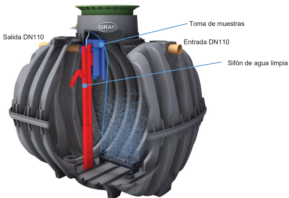
Imagen 2: Ejemplo de oneAdvanced 3-9 EW en un depósito Carat
