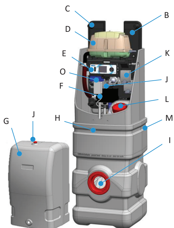
Imagen 6: Diseño técnico con el ejemplo de un armario de conexiones exterior M
