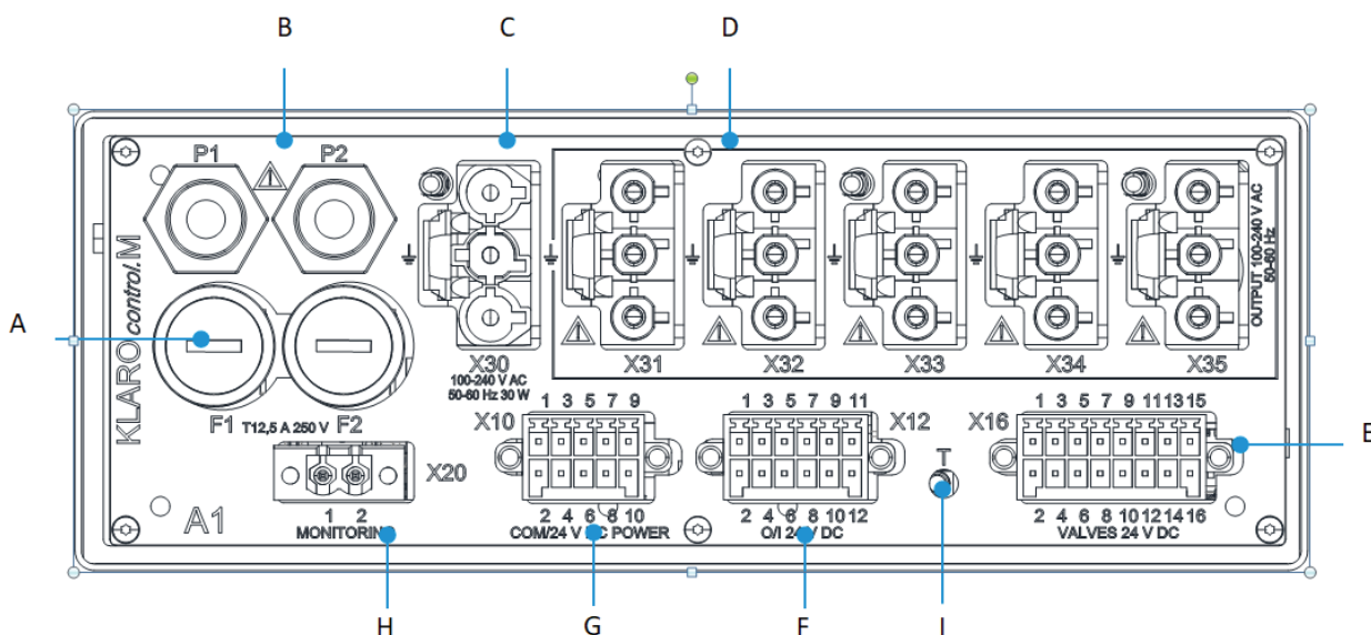
Imagen 15: Conexiones eléctricas KLcontrol.M
