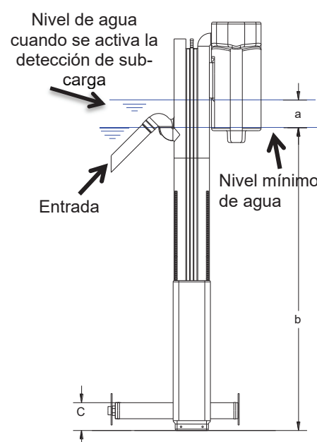
Imagen 13: Sifón de agua limpia, alturas en el reactor SBR
