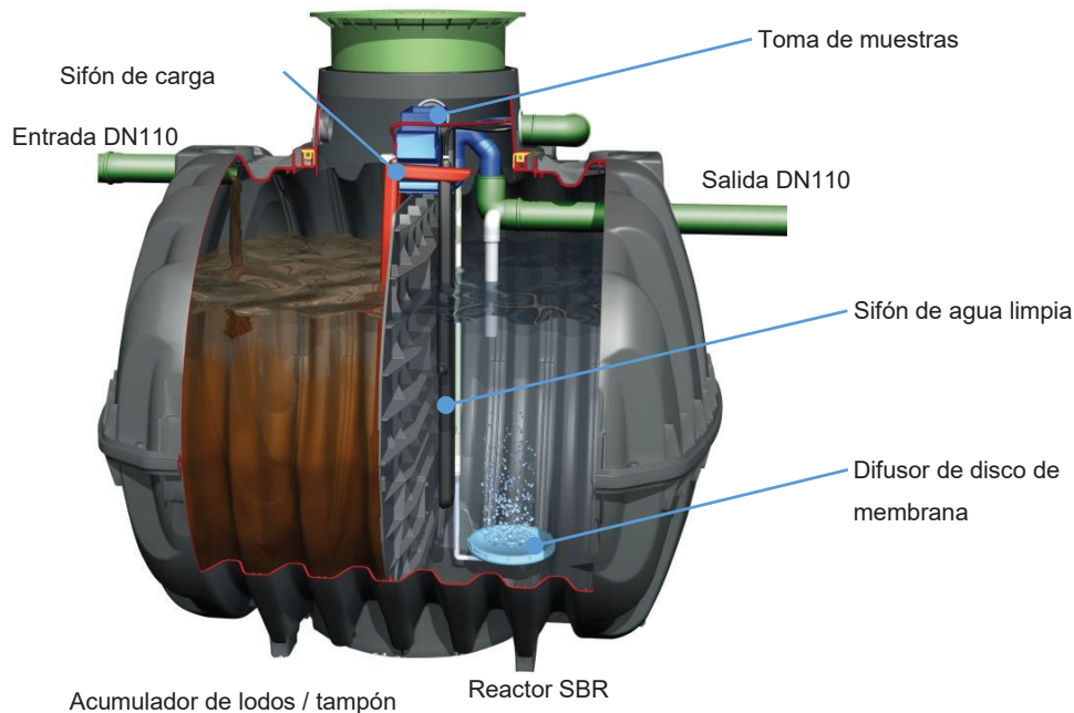
Imagen 3: Ejemplo de oneAdvanced 10-14 EW en un depósito Carat
